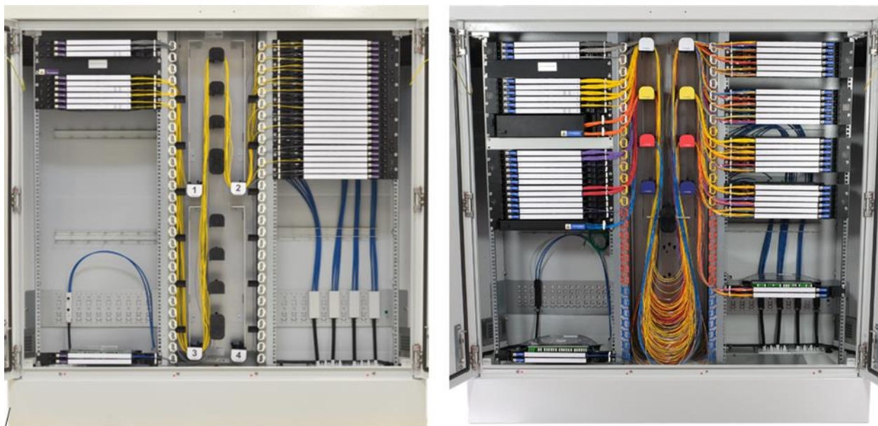
Exemples de PM avec 576 fibres distribuées, brassage en W et en M
