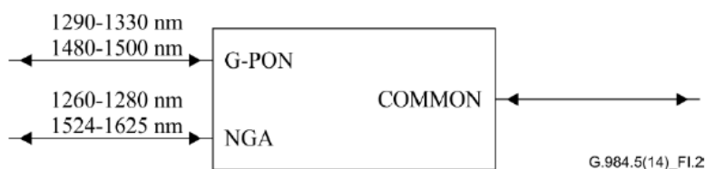
Cas WDM1r – Support GPON et XG(S)-PON
