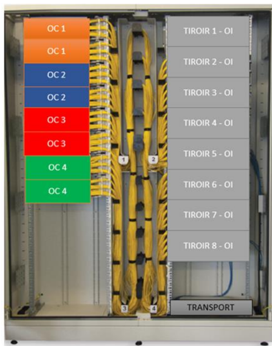
Armoires « Indoor » 2 x 40U avec zone de brassage en « W » ou « M » et tiroirs de distribution en 4U
