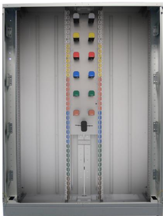
Armoires « Indoor » 2 x 40U avec zone de brassage en « W » ou « M » et tiroirs de distribution en 4U
