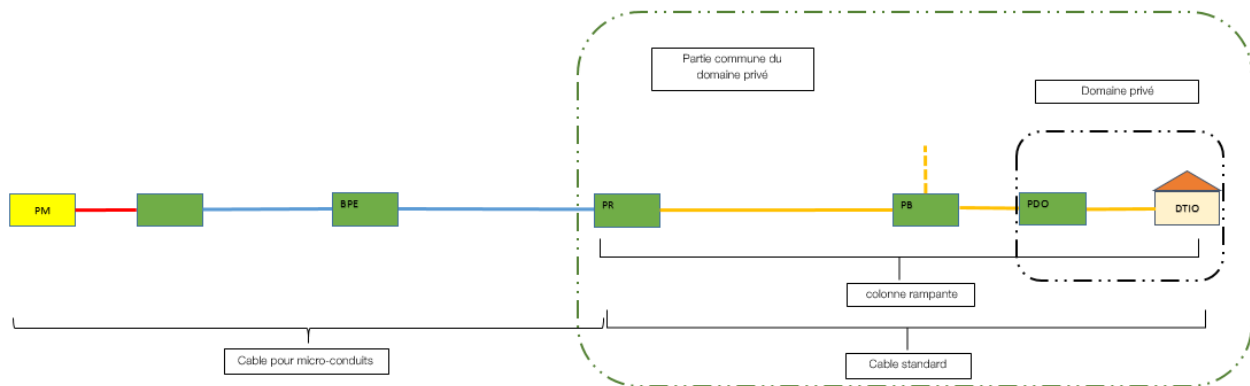
Figure 4 : Schéma de principe PM DTIO zone de logements individuels collectifs (lotissements)
