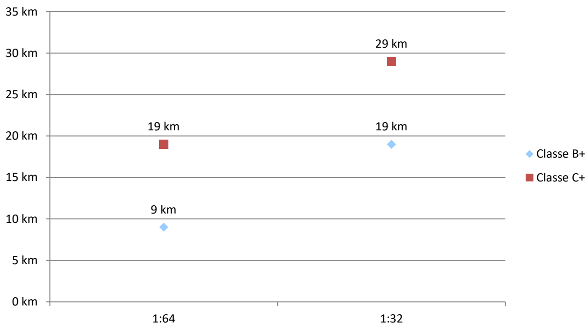
Distances disponibles en GPON en fonction de la configuration technique retenue
