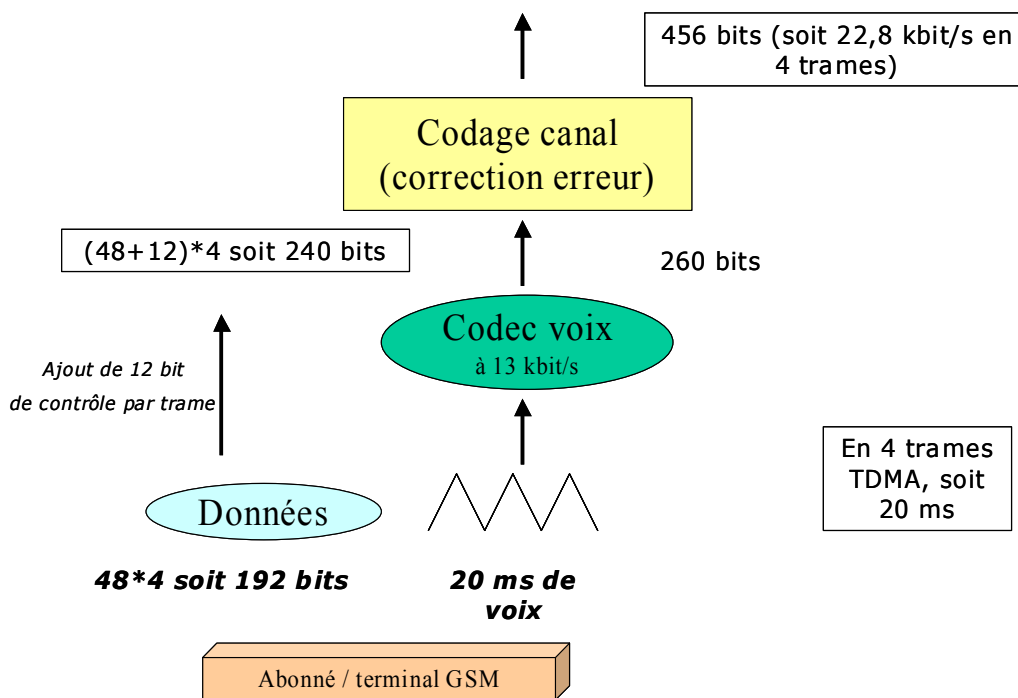
Transport de la voix et des données en mode circuit sur le réseau GSM
