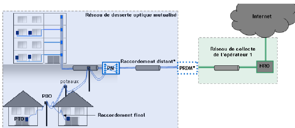
Architecture simplifiée d'un réseau FttH en dehors des zones très denses
